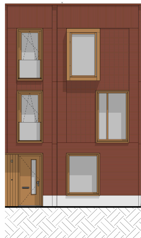
voorgevel 1 : 100
